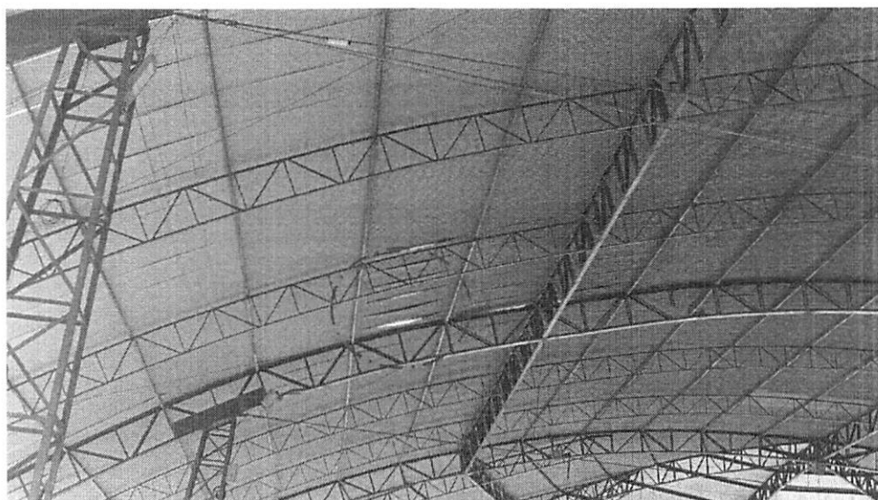
Foto 04 – Na imagem acima observa-se telhas amassadas em virtude da estrutura metálica que sustentam as telhas ter ser movimentado.
