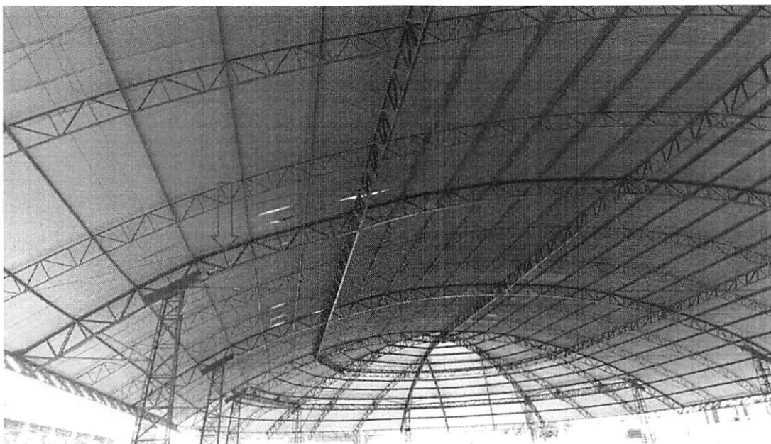
Foto 02 – Na imagem acima, é possível notar que o arco metálico está se movimentando no sentido que as setas indicam, ou seja, não se tem um arco perfeito. O que demonstra que a estrutura vem sofrendo movimentações ao longo do tempo.
