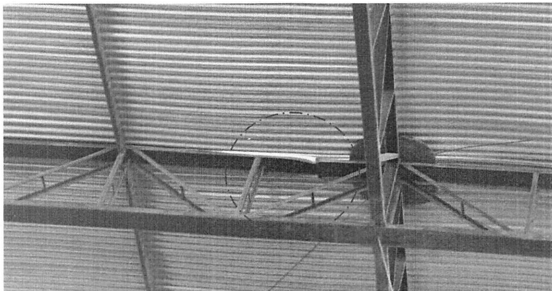
Foto 03 – Na imagem acima, podemos identificar que a estrutura do arco já está por sofrer rompimento.
