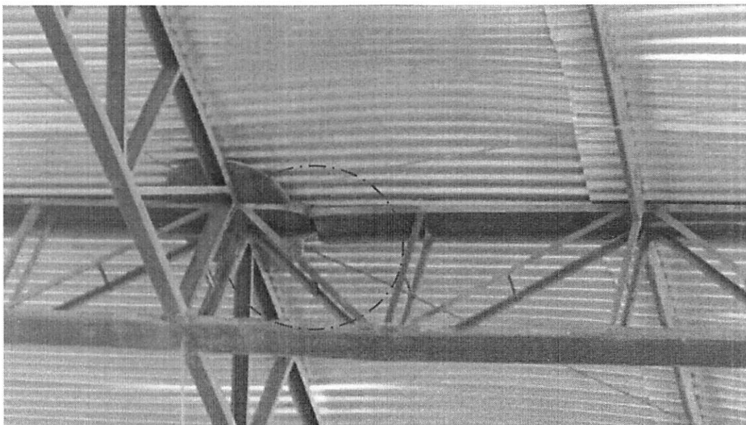
Foto 04 – Na imagem acima, Na imagem acima, podemos identificar que a estrutura do arco já está por sofrer rompimento.
